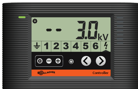
Il display mostra l'impostazione di fabbrica con l'allarme corrente disabilitato ed quello del voltaggio a 3.0KV
