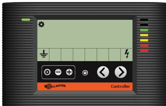
Kontrollenheten visar utgångsspänningen är justeras.
