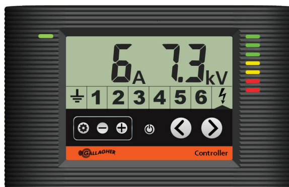
Kontrolleren viser, at spændingsgiveren fungerer normalt
