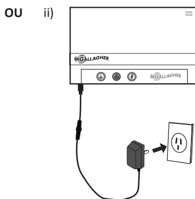
Adaptateur CC (G40132) secteur 110/230 volts CA
