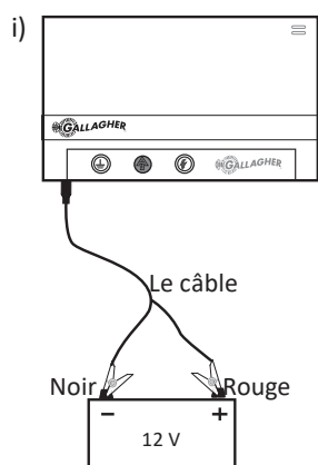
Batterie 12 volts via le câble
